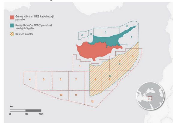
Şekil 4. MEB alanlarında kalan alanlar ve Türkiye'nin arama yaptığı hedeflediği ruhsatlar.
