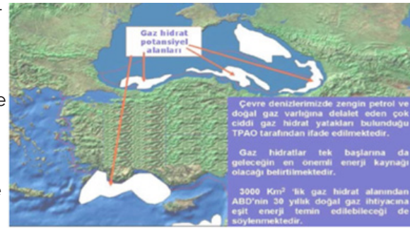
Şekil 2. Türkiye'nin çevreleyen denizlerdeki potansiyel gaz hidrat yataklarının konumları ( https://bau.edu.tr/haber/15966-dogu-akdeniz%25E2%2580%2599deki-hidrokarbon-rezervleri-turkiye%25E2%2580%2599nin-572-yillik-ihityacini-karsiliyor#_ftn1 )
