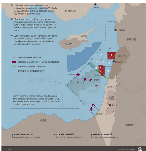
Şekil 3. Havzadaki ruhsat alanları ve keşif alanları (AA, 2019'dan değiştirilerek).
